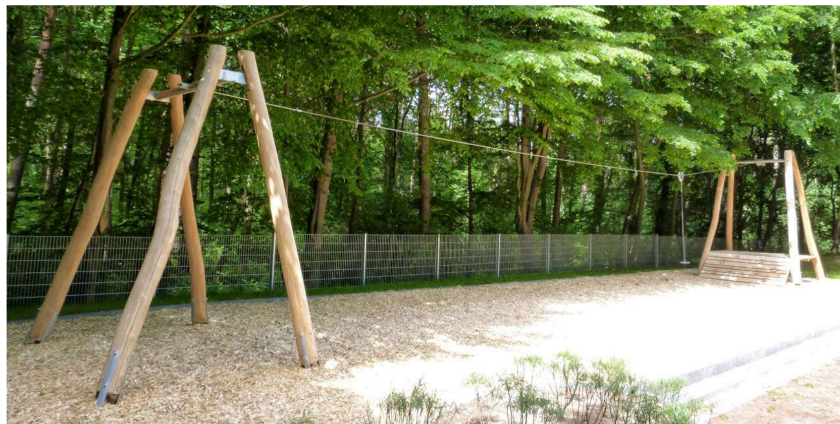
Tyrolienne 25 m Longueur de la zone de glisse : 25 m Longueur totale (avec plateforme et zone de sécurité) : 30,5 m
